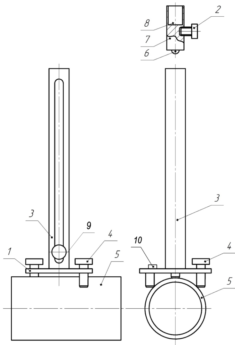
1 – основание; 2 – винт-рукоятка; 3 – направляющая; 4 – винты-ножки; 5 – труба с испытуемым покрытием; 6 – стальной боек; 7 – груз; 8 – утяжелитель; 9 – «0» шкалы; 10 – уровень.
